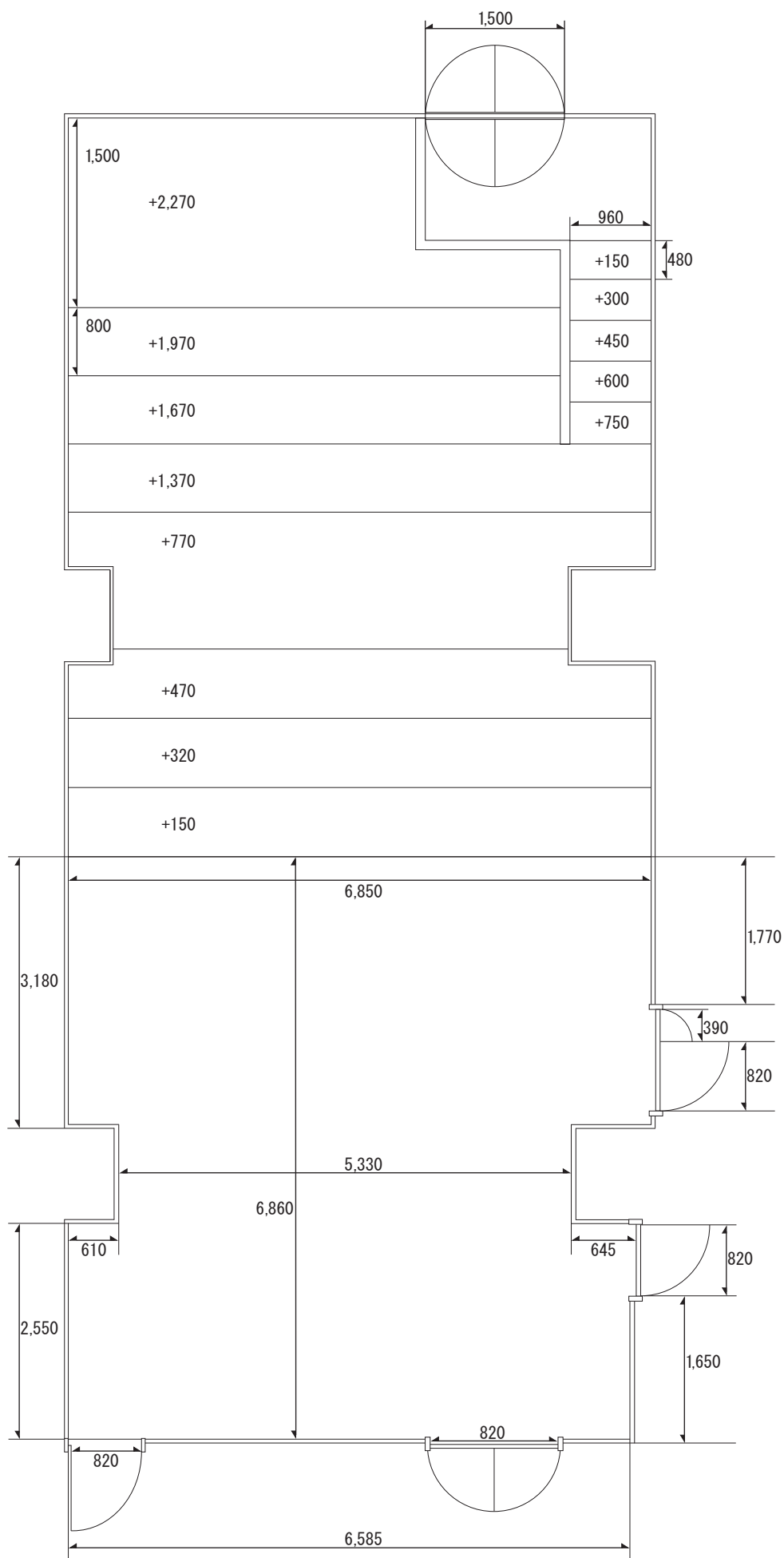
シアターZOO mm寸法図
